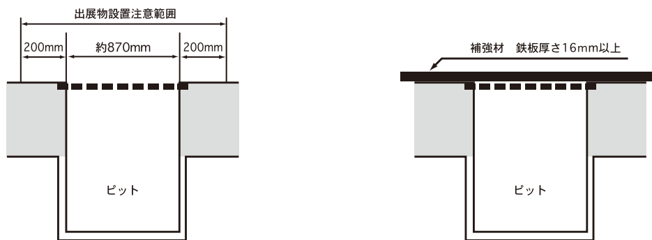
ピット周辺図
