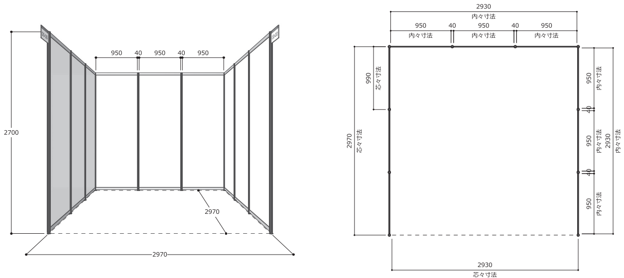
システムパネル壁面形状
