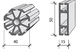
◆ポール断面図
